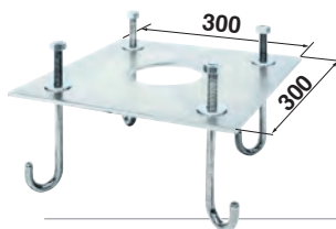
ACG8110 PIASTRA DI FISSAGGIO da interrare
